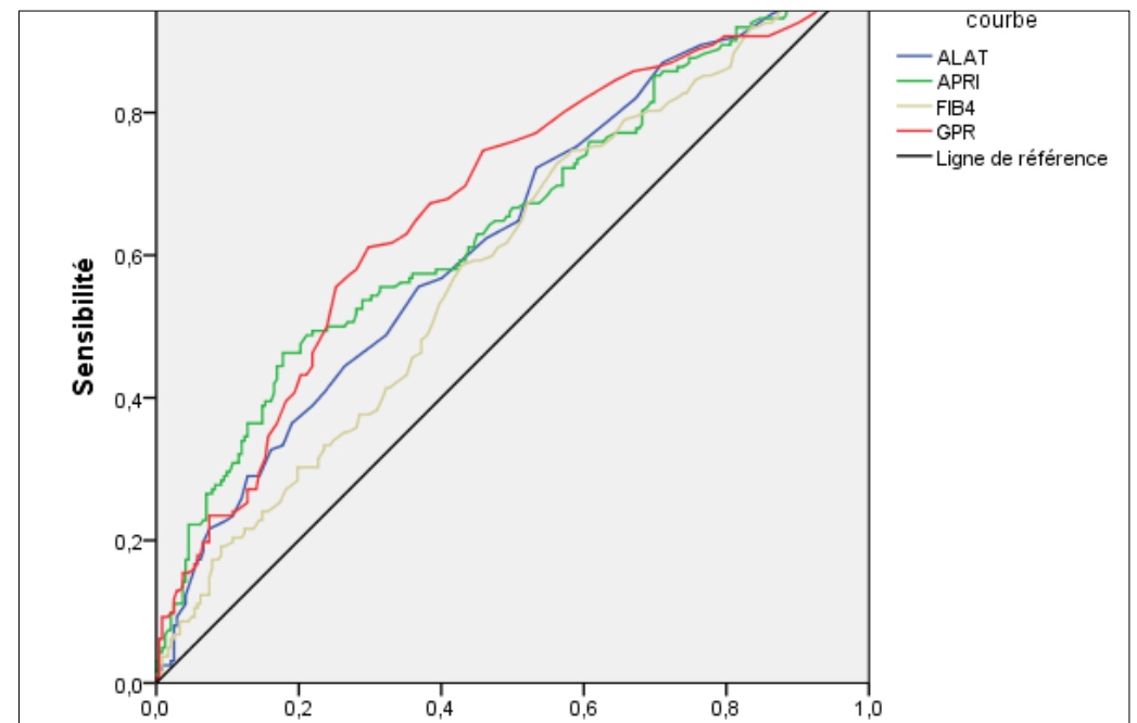
Figure 1 : Courbe ROC des 3 scores biologiques
